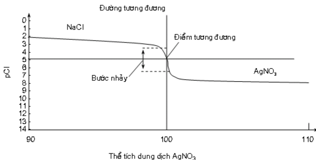
Hình 9.2. Đường cong chuẩn độ dung dịch \text{NaCl} 0,1N bằng dung dịch \text{AgCl} 0,1N
