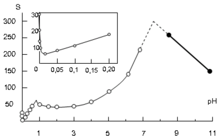
Hình 10.1. Sự phụ thuộc của độ tan EDTA (trong 100 ml nước) và pH ở 20^\circ\text{C}
