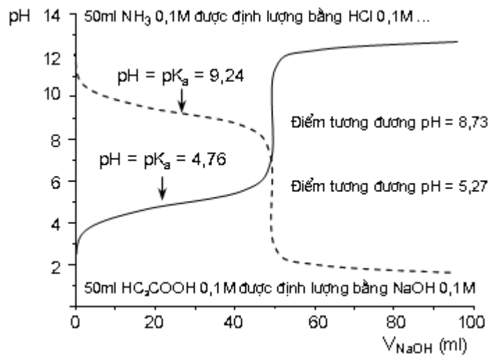
Hình 7.20. Trung hoà base yếu (0,1N) bằng acid mạnh (c) và ngược lại
