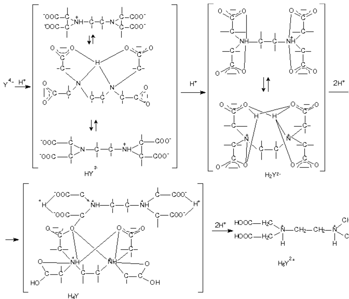
Hình 10.2. Sơ đồ trao đổi proton của anion Y^{4-}
