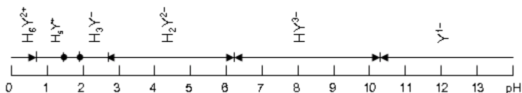
Hình 10.3. Biểu đồ vùng tạo thành những dạng khác nhau của EDTA
