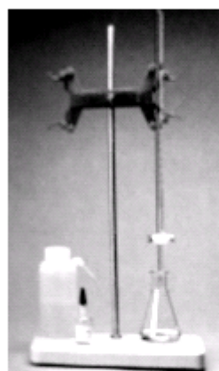
Hình 8.2. Phản ứng oxy hoá – khử xảy ra trong một dung dịch
