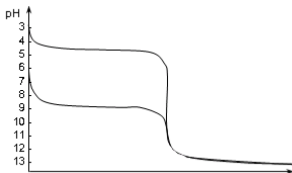
Hình 7.26. Chuẩn độ chỉ acid boric (1) và chuẩn độ acid boric khi có mặt mannitol (2)
