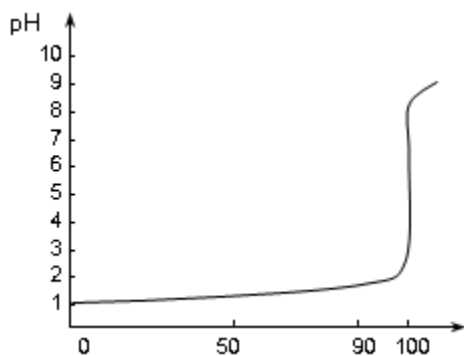
Hình 7.21. Đường cong chuẩn độ khi trung hoà 1 acid mạnh bằng 1 base yếu
