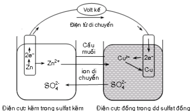
Hình 8.4. Sơ đồ cấu tạo 1 pin điện hoá
