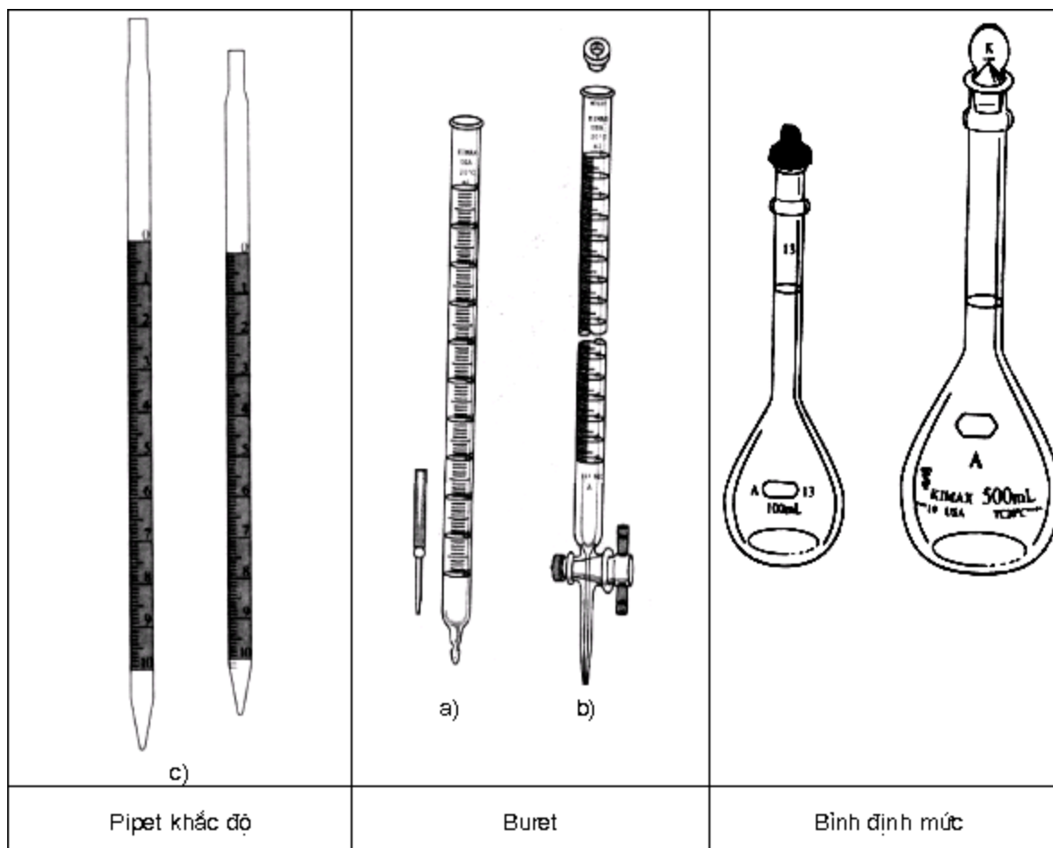
Hình 6.1. Một số dụng cụ sử dụng trong chuẩn độ thể tích
