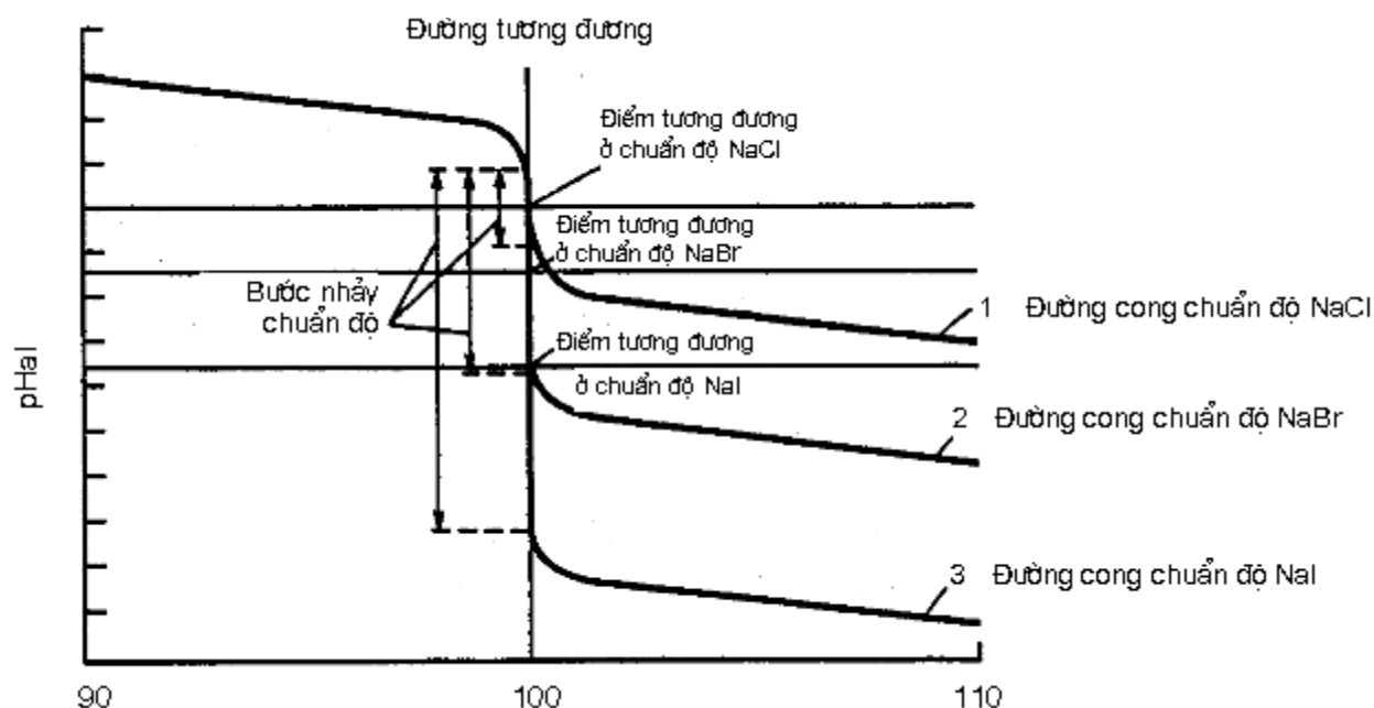
Hình 9.4. Ảnh hưởng giá trị độ tan của chất kết tủa tách ra đến bước nhảy chuẩn độ
