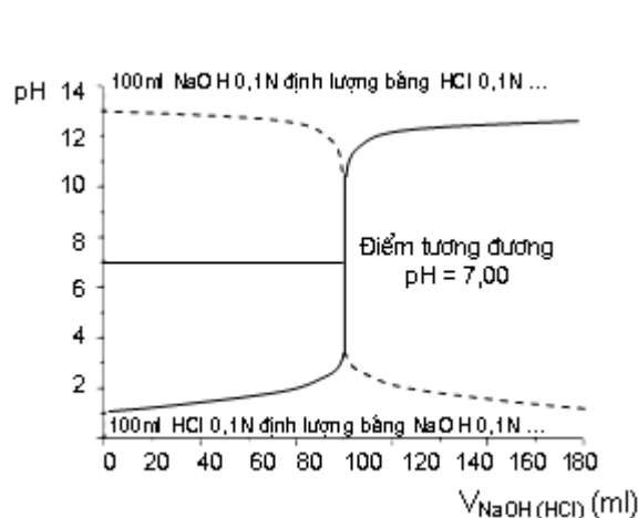
Hình 7.14. Trung hoà acid mạnh (0,1N) bằng base mạnh (0,1N) hoặc ngược lại
