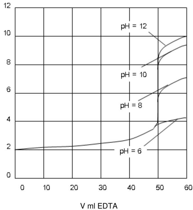
Hình 10.6. Ảnh hưởng của pH đến chuẩn độ của dung dịch \text{Ca}^{2+} 0,0100 M bằng dung dịch EDTA 0,0100M
