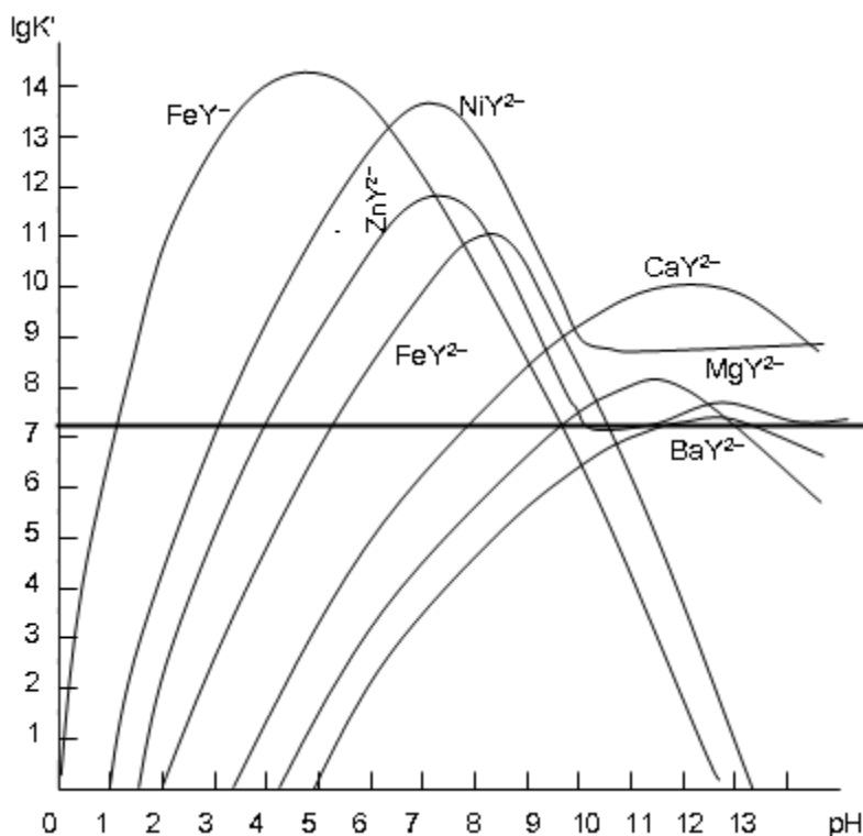
Hình 10.5. Sự phụ thuộc hằng số bền điều kiện của một số phức vào pH (tổng nồng độ [\text{NH}_3] + [\text{NH}_4^+] = 1,0\text{M} )
