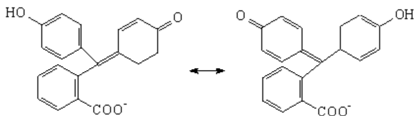
Hình 7.7. Dạng quinon của phtalein có màu trong môi trường kiềm (b,c,d)
