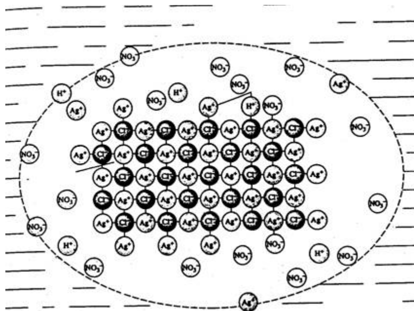
Hình 9.6. Cấu tạo hạt keo AgCl trong dung dịch AgNO 3
